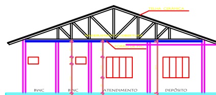
CORTE A Escala 1/100
