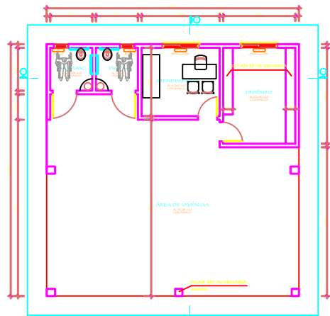
PLANTA BAIXA Escala 1/100
