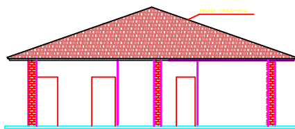
FACHADA Escala 1/100
