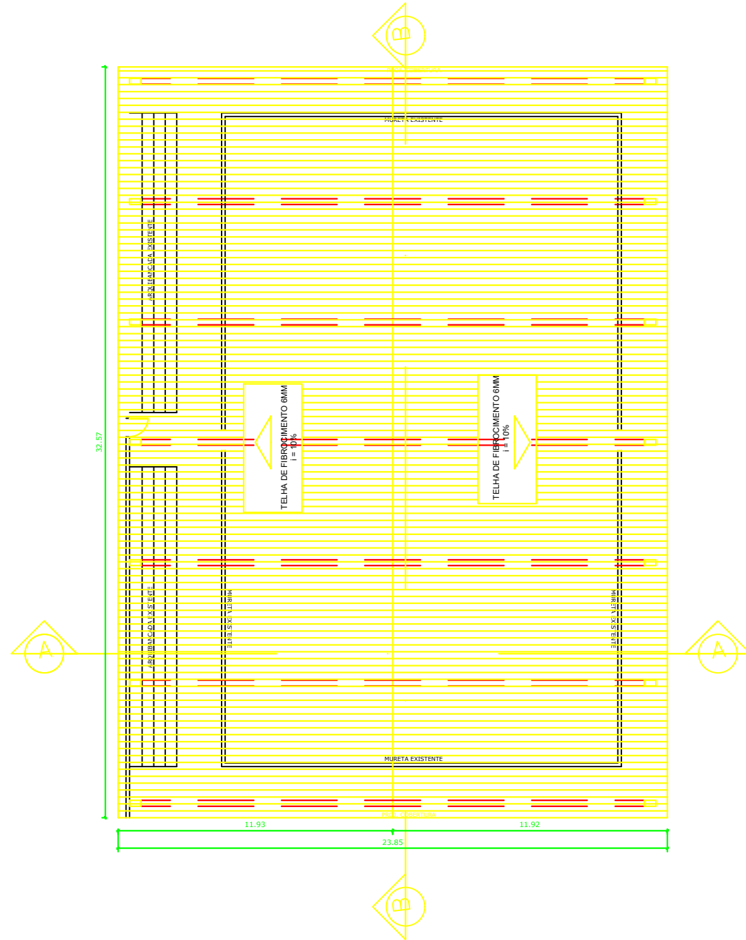
PLANTA DE COBERTURA ESCALA 1/100
